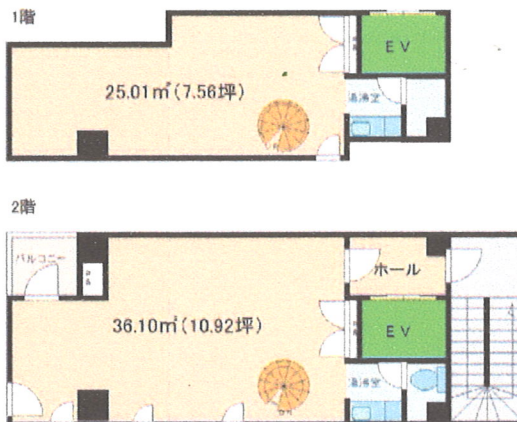
間取図(平面図)
